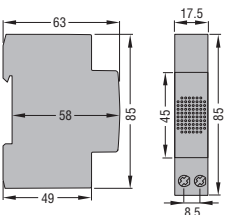
MODULARE SICHERHEITSTRANSFORMATOREN CTRS15VA - CTRS25VA
