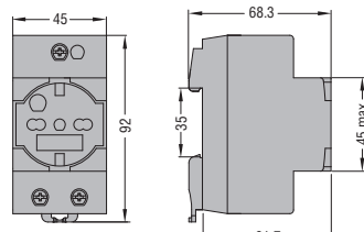
MODULARE STECKDOSE P1X7
