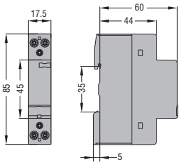
INSTALLATIONSSCHÜTZE CN20... - CN32... (1-polig - 2-polig)
