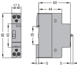
ANBAUBLÖCKE UND ZUBEHÖR Hilfskontakte CNH... - CNBX...
