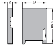
Distanzstück CNX80
