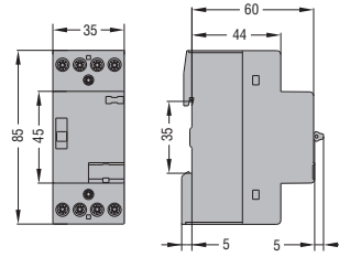
INSTALLATIONSSCHÜTZE MIT MANUELLER BETÄTIGUNG CNM20... - CNM32... (1-polig - 2-polig) CNM32... (3-polig - 4-polig)
